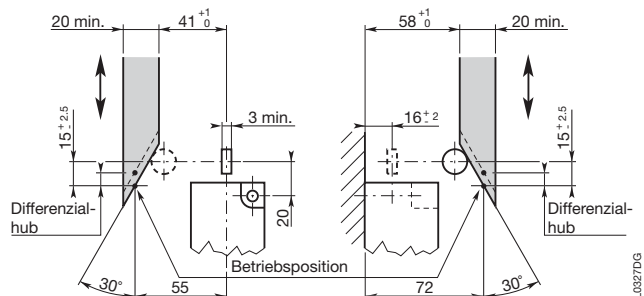
Form G seitliche Betätiger mit Rollendruckbolzen – seitliche Auslösung
