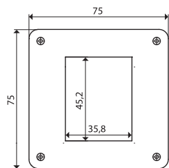
pohled shora
