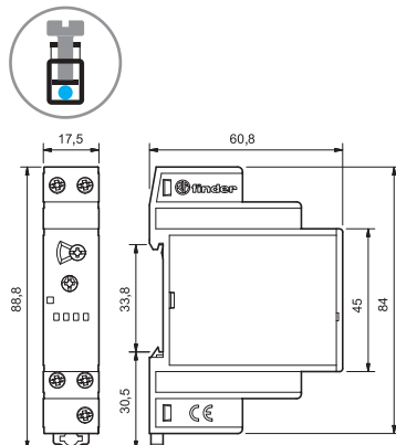
80.91 šroubové svorky
