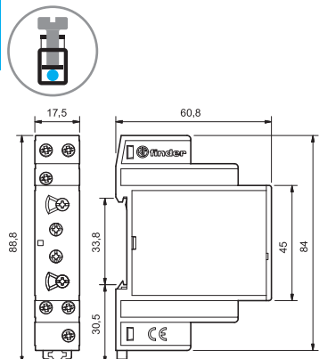
80.61 šroubové svorky
