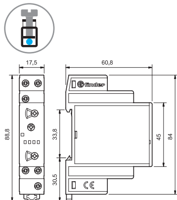
80.21 šroubové svorky
